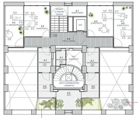
Planta Altell
