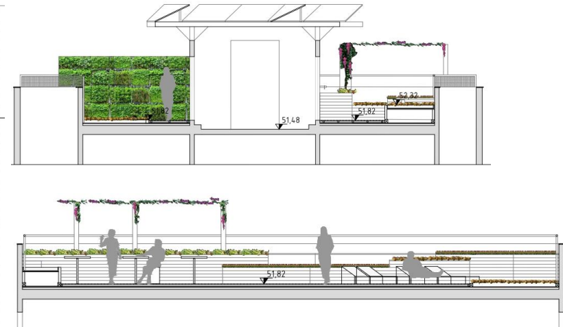
Seccions
