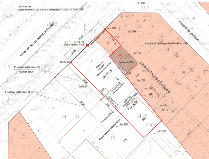
DETTALL COSSOS SORTINTS I TERRASSES (P1 I P2)
