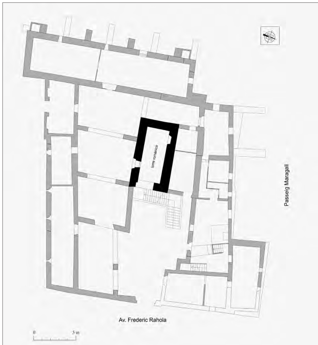
Planta general de la masia de Can Fargas. Realització: BAMMP Arquitectes i Associats
