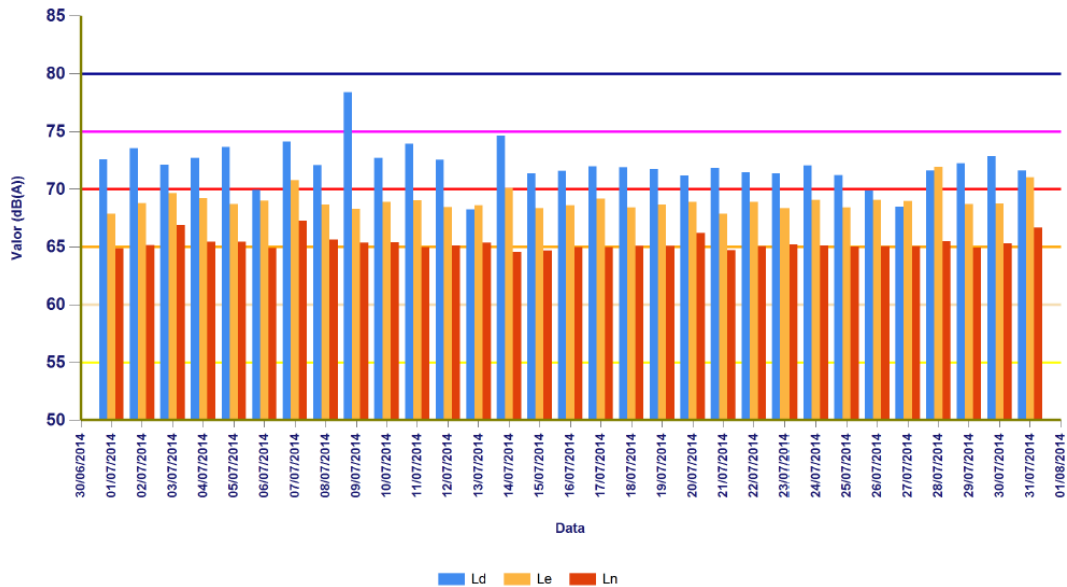
SENSOR: SA02 01/07/2014 - 31/07/2014
