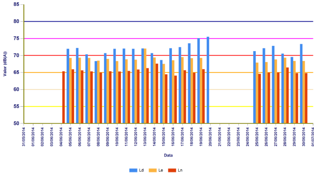
SENSOR: SA02 01/06/2014 - 30/06/2014
