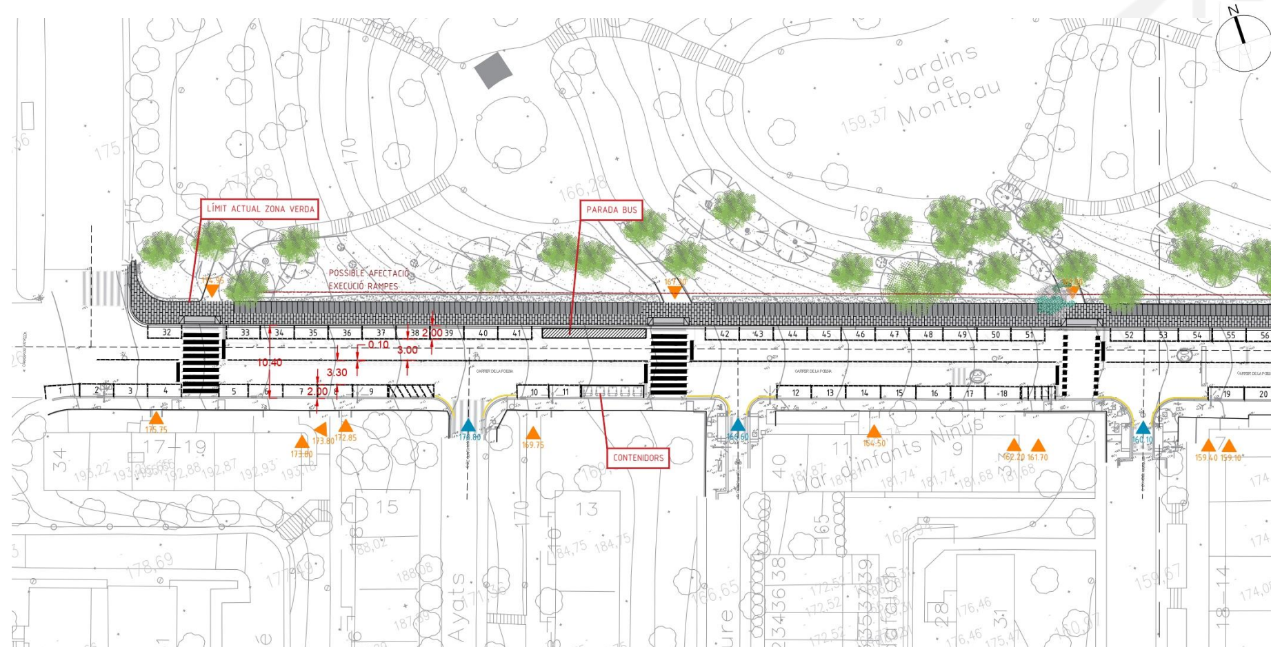
Planta proposta tram superior carrer de la Poesia.
