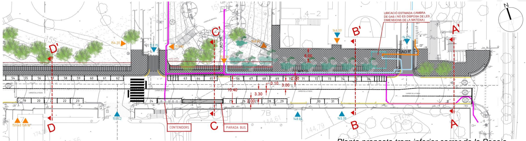
Planta proposta tram inferior carrer de la Poesia.
