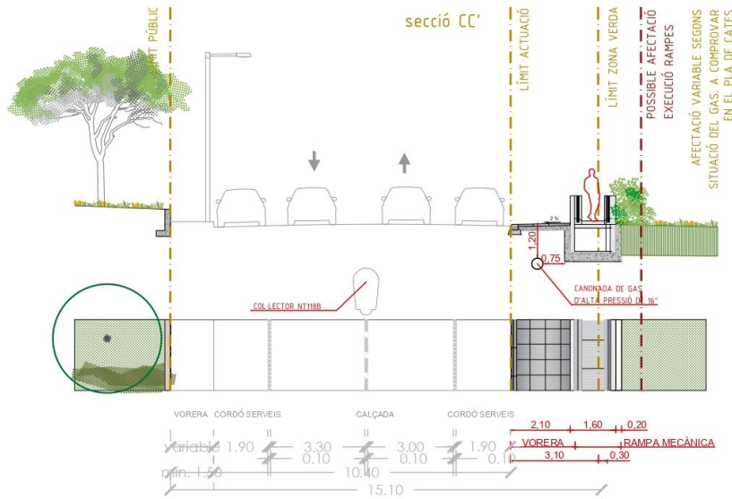
Secció del carrer de la Poesia, C-C'
