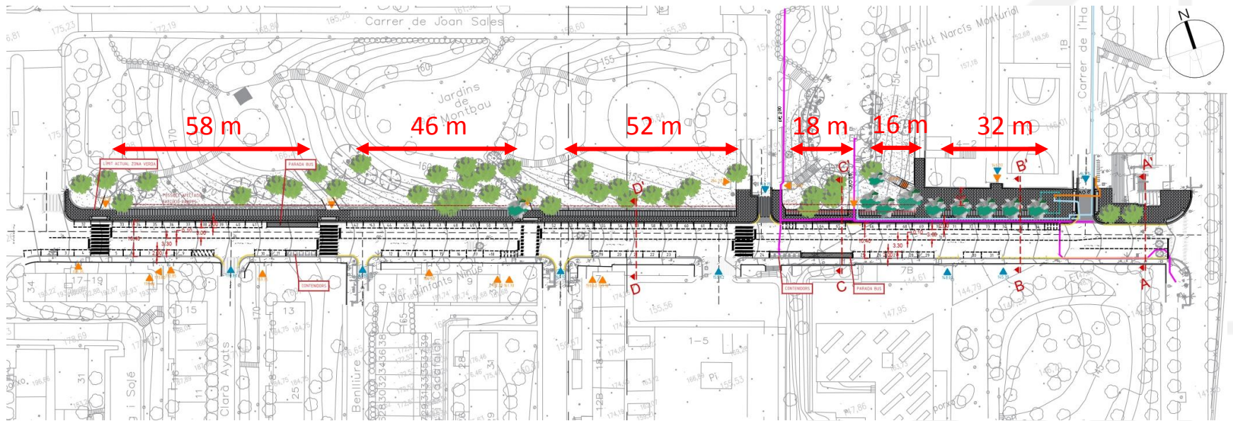
Planta proposta amb les longituds de les rampes mecàniques.
