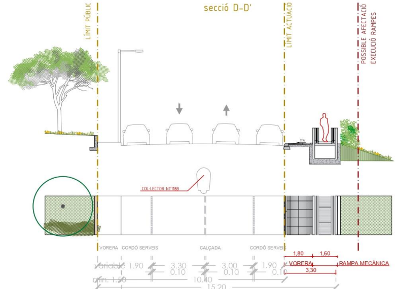
Secció del carrer de la Poesia, D-D'
