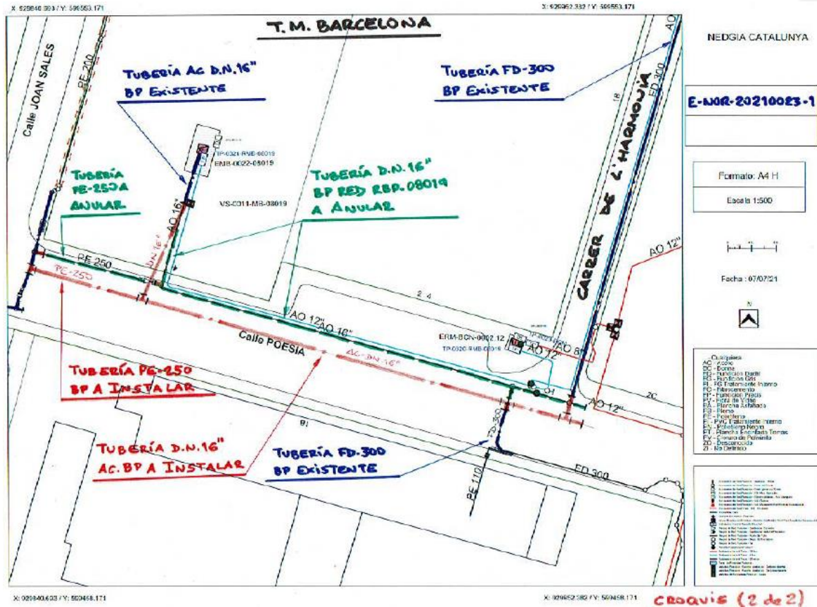
Esquema proposta desviament de gas segons assessorament de la companyia. NEDGIA Catalunya.
