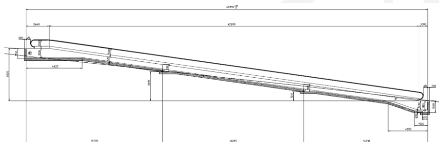
Esquema d'un tram de rampa mecànica.
