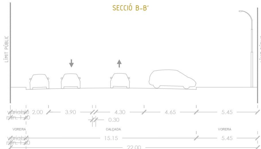
Secció actual del carrer, altura institut.
