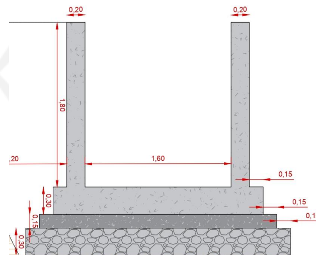
Secció esquemàtica del fossat de les rampes.
