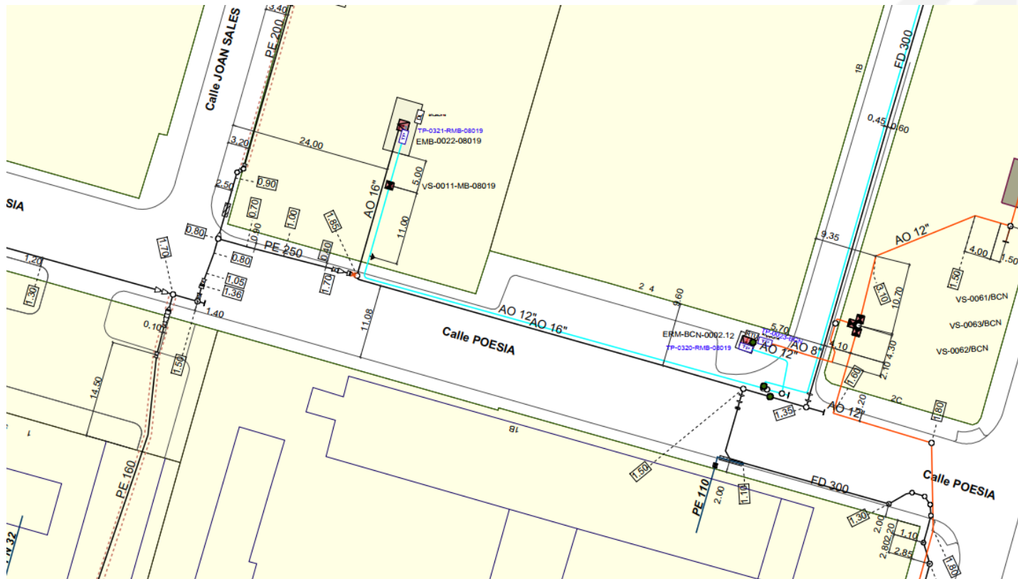
Planta del servei existent de gas (AsBuilt). NEDGIA Catalunya.
