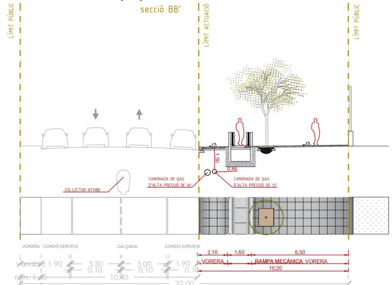
Secció del carrer de la Poesia, B-B'
