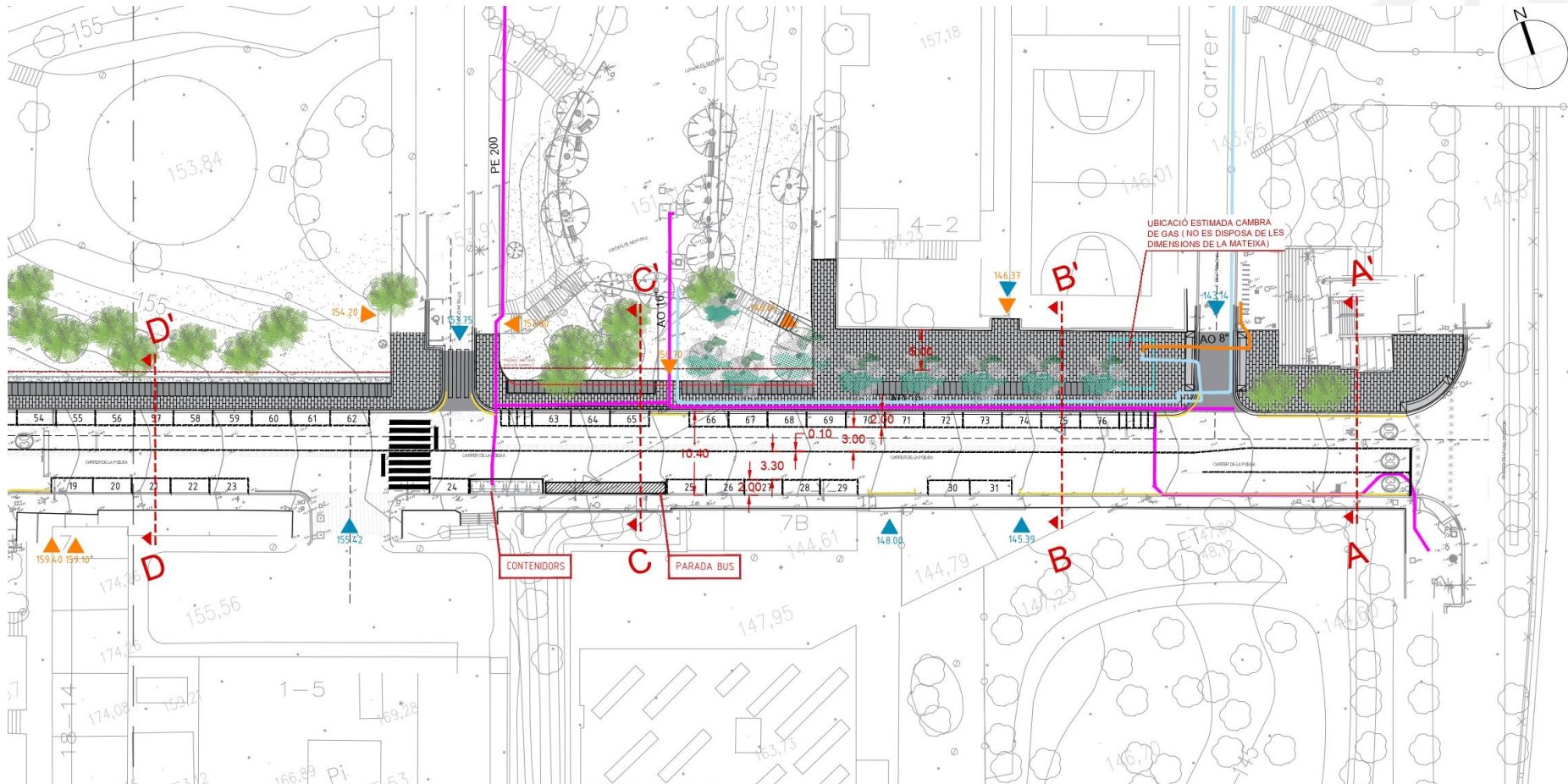
Planta proposta tram inferior carrer de la Poesia.
