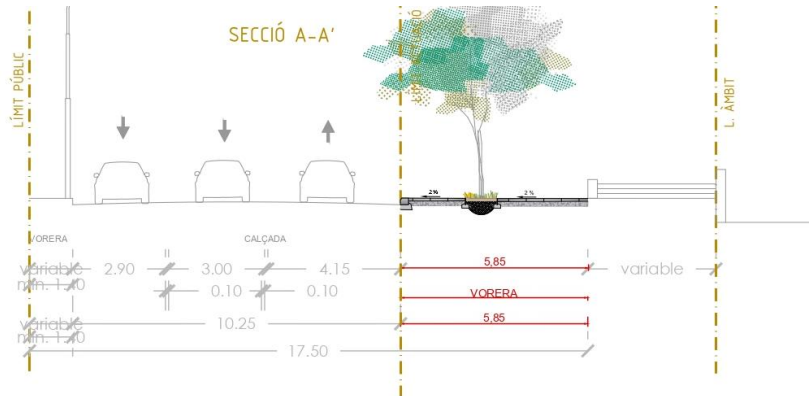
Secció del carrer de la Poesia, A-A'
