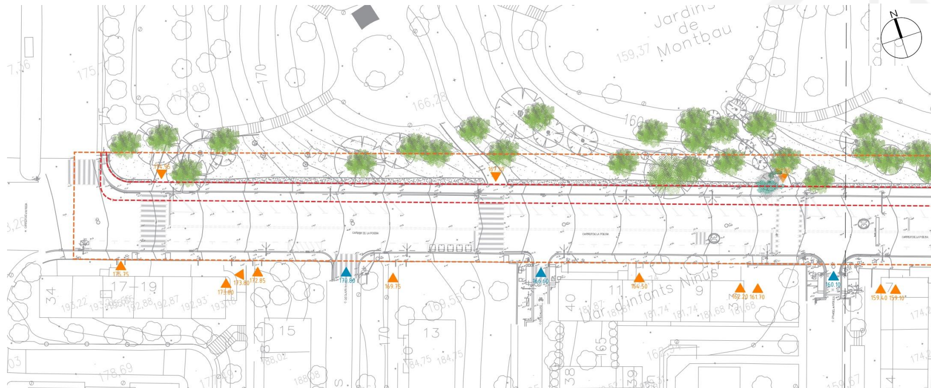
Planta estat actual detall del carrer de la Poesia
