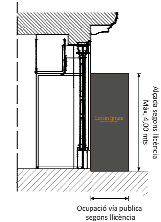
SECCIÓ TANCAMENT D'OBRA SOBRE VÍA PÚBLICA
