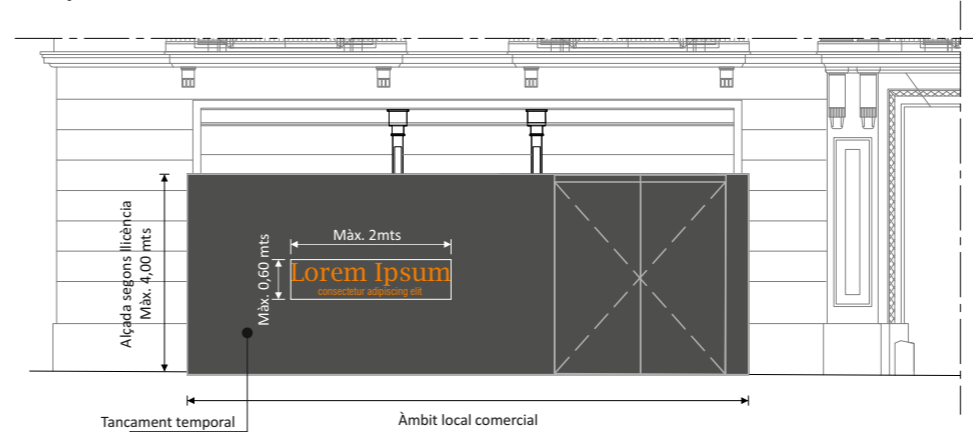
ALÇAT TANCAMENT D'OBRA SOBRE VÍA PÚBLICA
