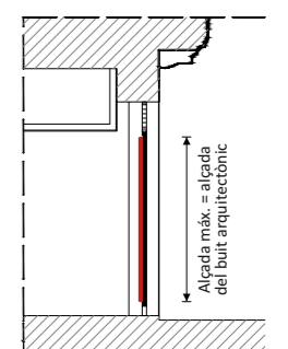
SECCIÓ DEL TANCAMENT DELS BUITS
