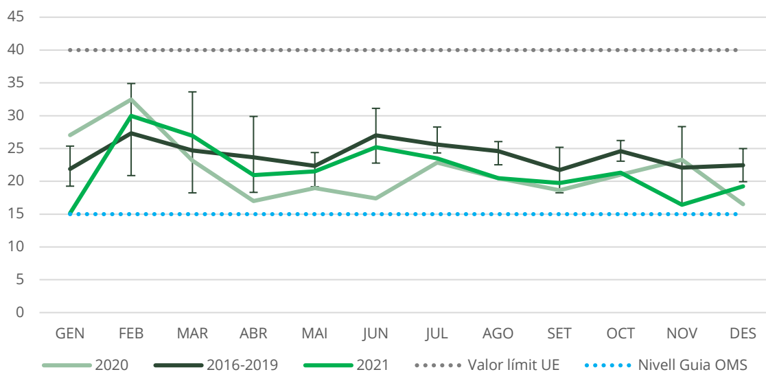
Figura 11. Mitjana mensual agregada a les estacions de fons urbà de PM 10 (en µg/m 3 ) per als anys 2020 i 2021 i per al període 2016-2019. (Dades mètode gravimètric)
