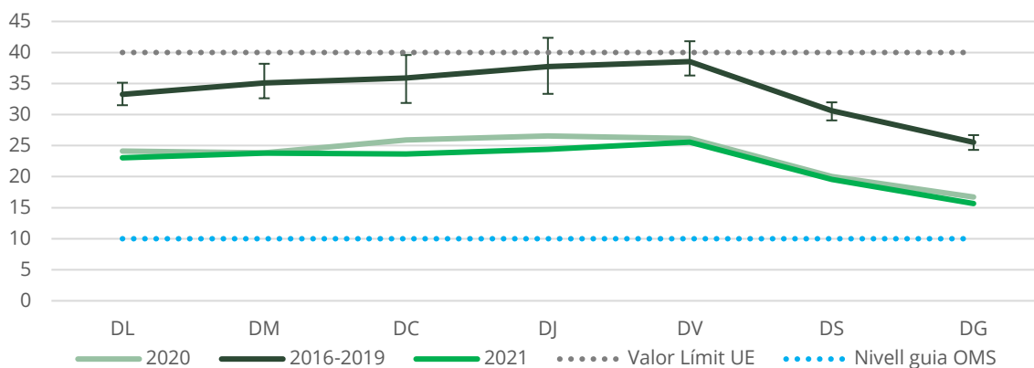
Figura 7. Mitjana diària agregada per estacions de fons urbà de NO 2 (en µg/m 3 ) per als anys 2020 i 2021 i per al període 2016-2019.
