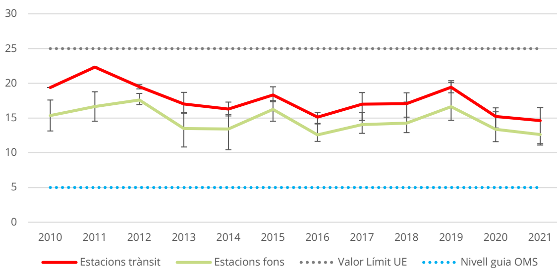
Figura 17. Evolució temporal de la mitjana anual agregada per estacions de trànsit i de fons de PM_{2,5} (en \mu\text{g}/\text{m}^3 ) pel període 2010-2021. (Dades mètode gravimètric)
