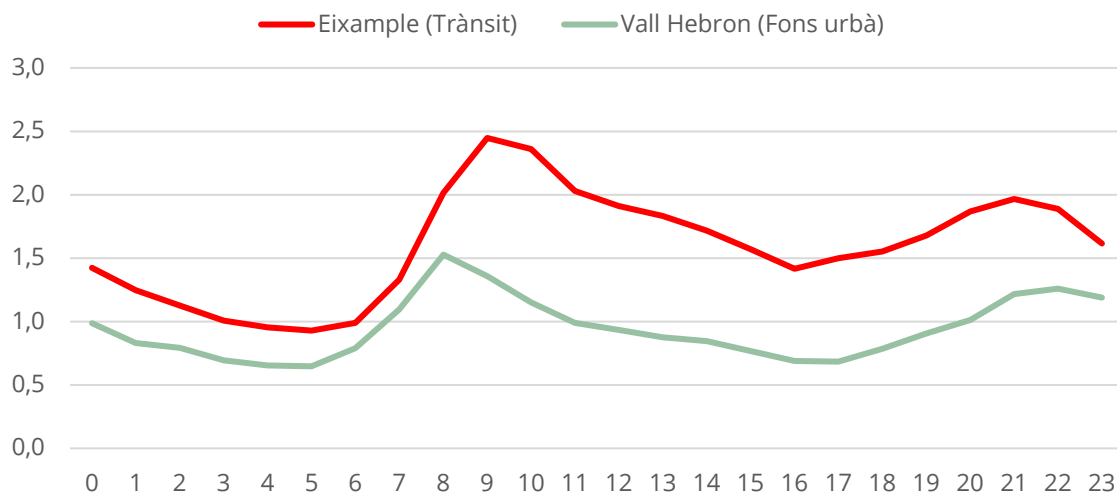
Figura 23. Mitjana horària per estacions de carboni negre (en \mu\text{g}/\text{m}^3 ) per a l'any 2021.
