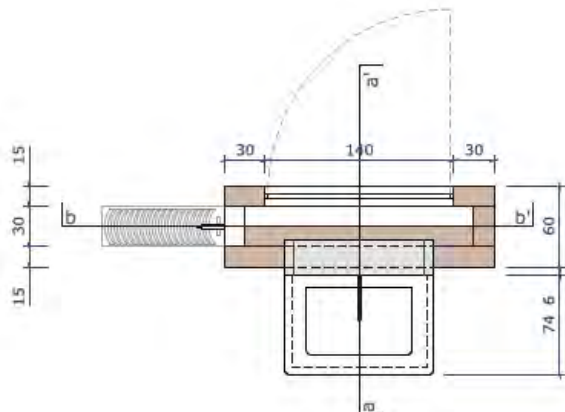
Planta 1 - 1'
