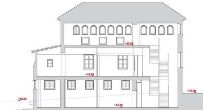
SECCIÓ 1-1'
