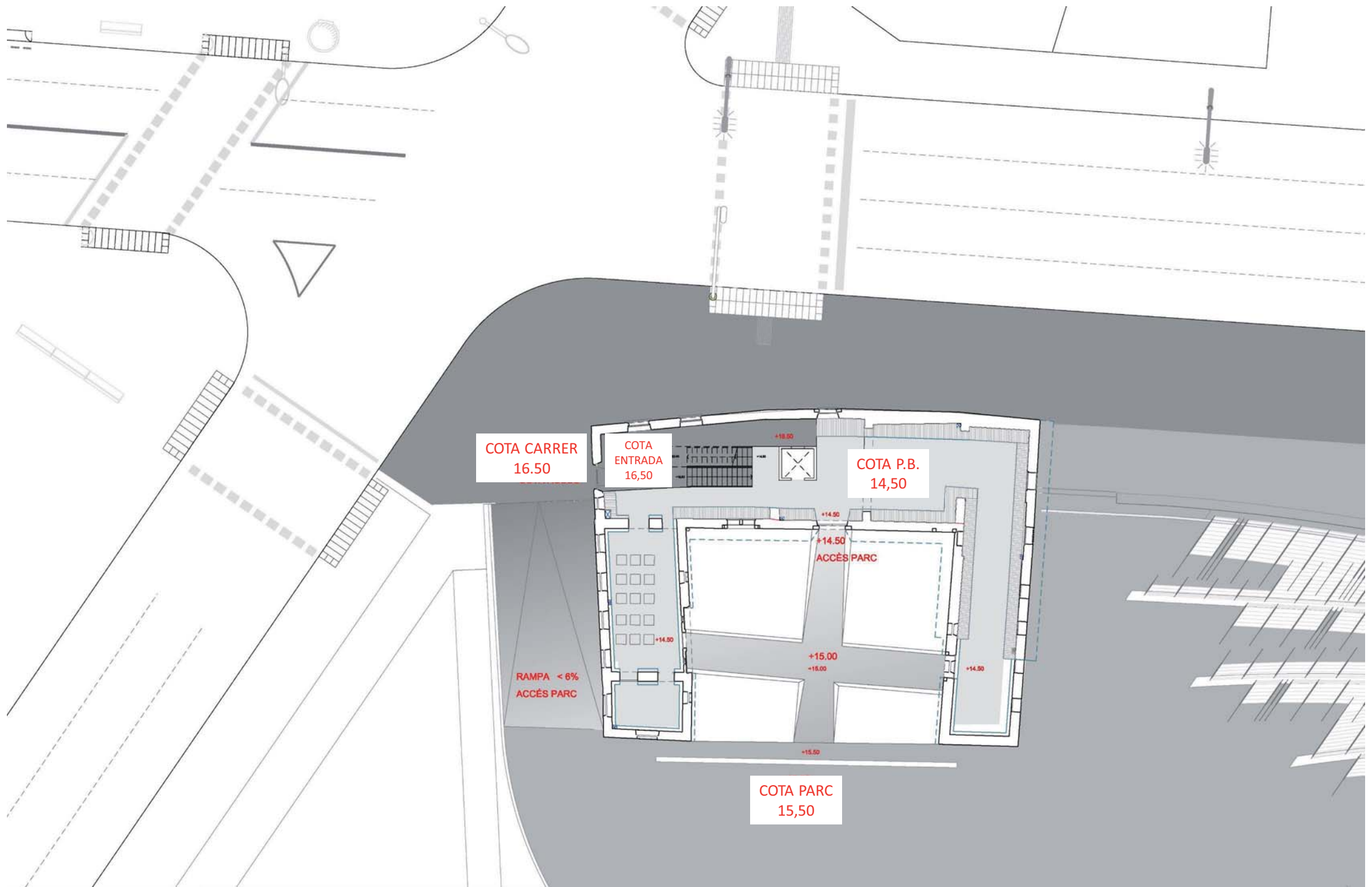
COTA DEL CARRER I ACCÉS (16.50). COTA DE PARC (15.50). COTA DE LA PLANTA BAIXA (ORIGINAL 14.50)
