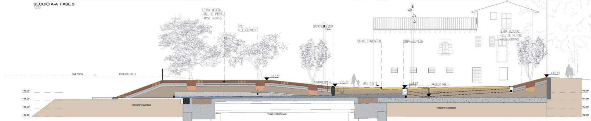
SECCIÓ A-A FASE 2 1:200
