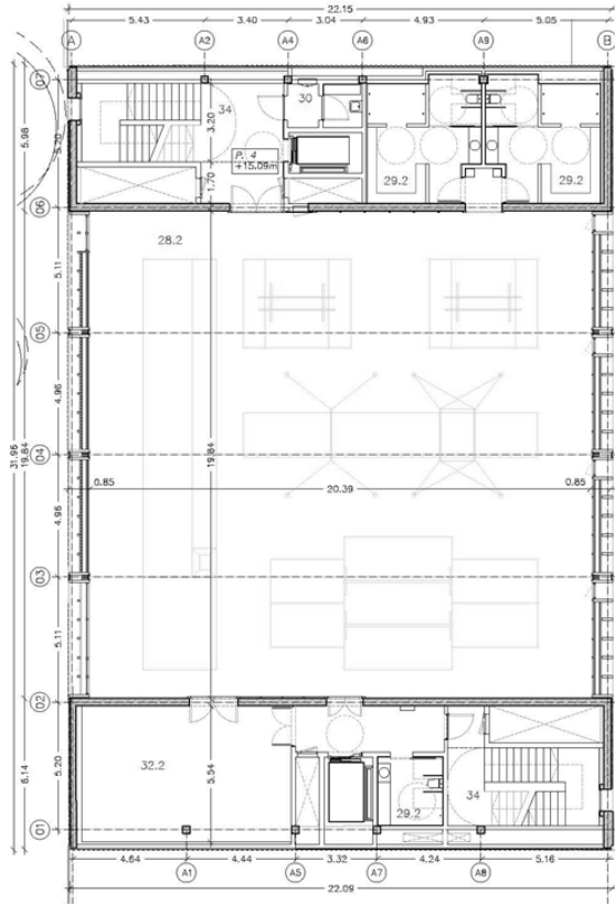
PLANTA QUARTA
