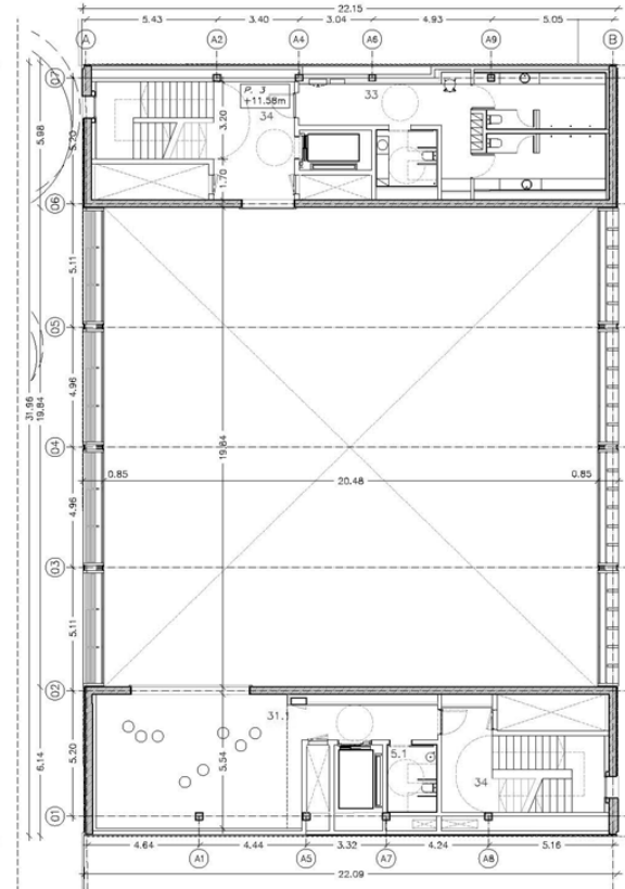
PLANTA TERCERA
