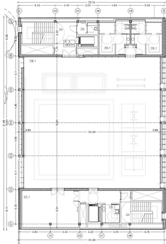
PLANTA SEGONA
