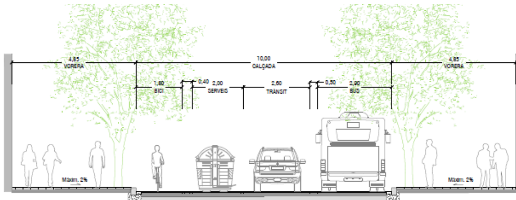
TRAM ENTRE C/ VALÈNCIA I C/ MALLORCA SECCIÓ PROPOSTA
