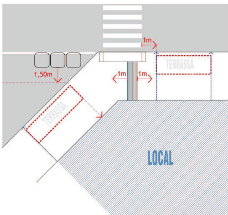
TERRASSES A CALÇADA
