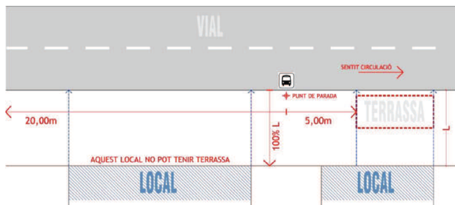
Punt de parada sense marquesina
